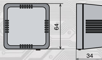
Snímač do interiéru - P10M
