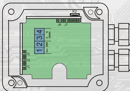
K2... konektor USB mini B
