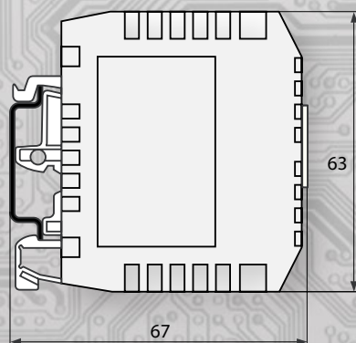
Uchytení na lištu dle EN 50 022 – 35 x 7,5
