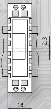
Uchytení na lištu dle EN 50 022 – 35 x 7,5
