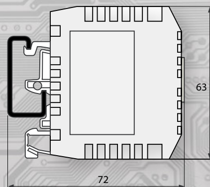
Uchytení na lištu G dle EN 50 035 – G32
